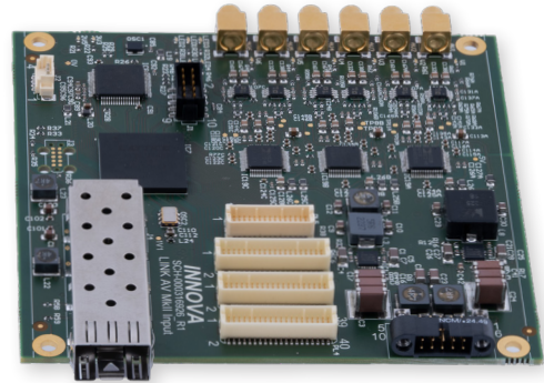
AV 6 ch. Input
